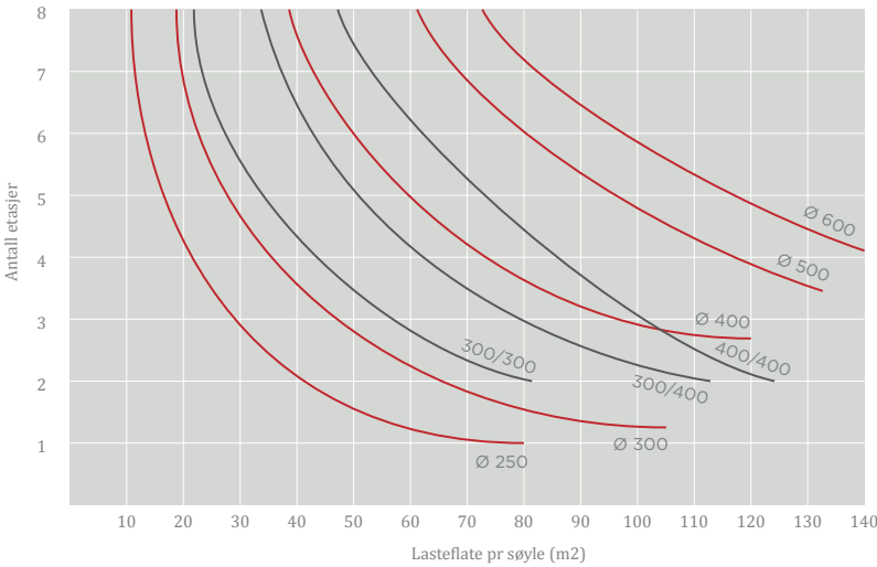
Orienterende bæreevne søyler, fleretasjesbygg
